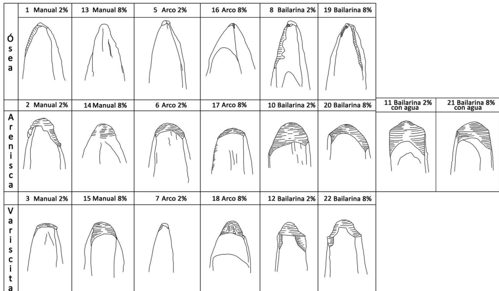
Fig. 1.—Perfiles de los punzones de metal después del uso.
